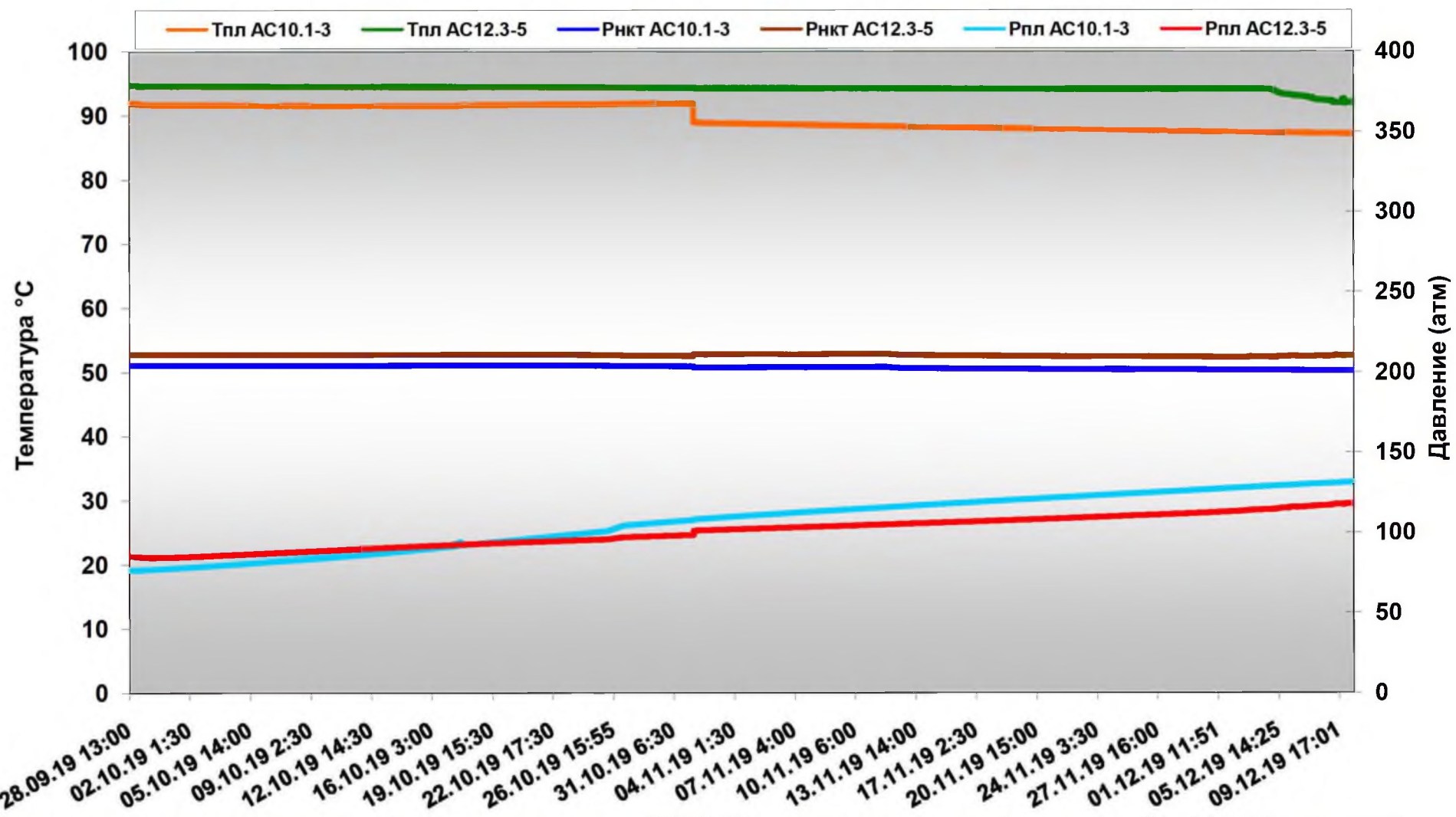
Двухпакерная компоновка с глубинным комплексом ИСДК-2G с замером давлений в режиме "on-Line" (пьезометр) с 13ч00м 28.09.19г. по 18ч27м 29.12.19г.
