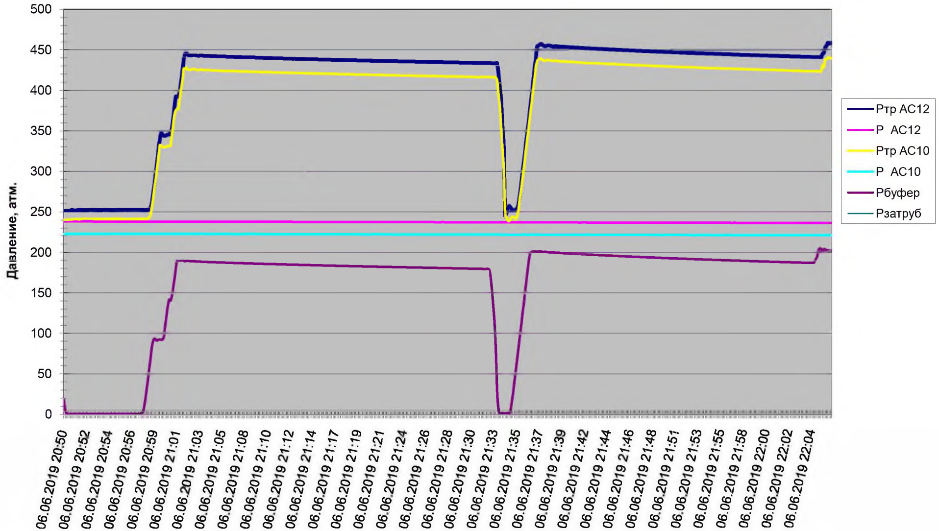
Диаграмма опрессовки лифта НКТ скважины в режиме реального времени
