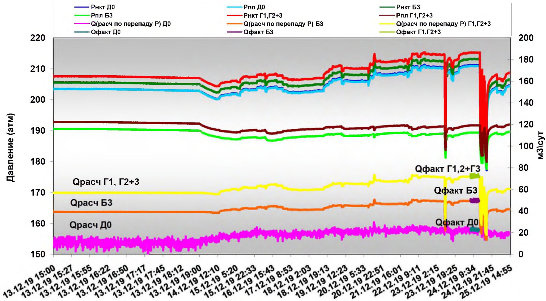
Трехпакерная компоновка с глубинным комплексом ИСДК-2G с замером давлений в режиме "on-Line" с 15ч00м 13.12.19г. по 15ч05м 25.12.19г.
