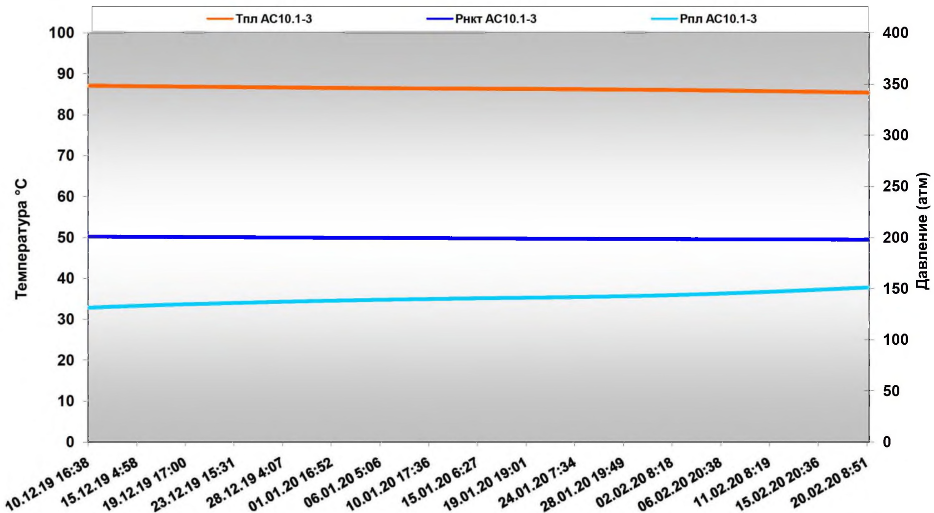
Данные с глубинного комплекса ИСДК-2С с замером давлений в режиме "on-Line" с 10.12.2019г. по 20.02.2020г. (в пьезометрической скважине между пространством в НКТ и интервалом перфорации нет сообщения)
