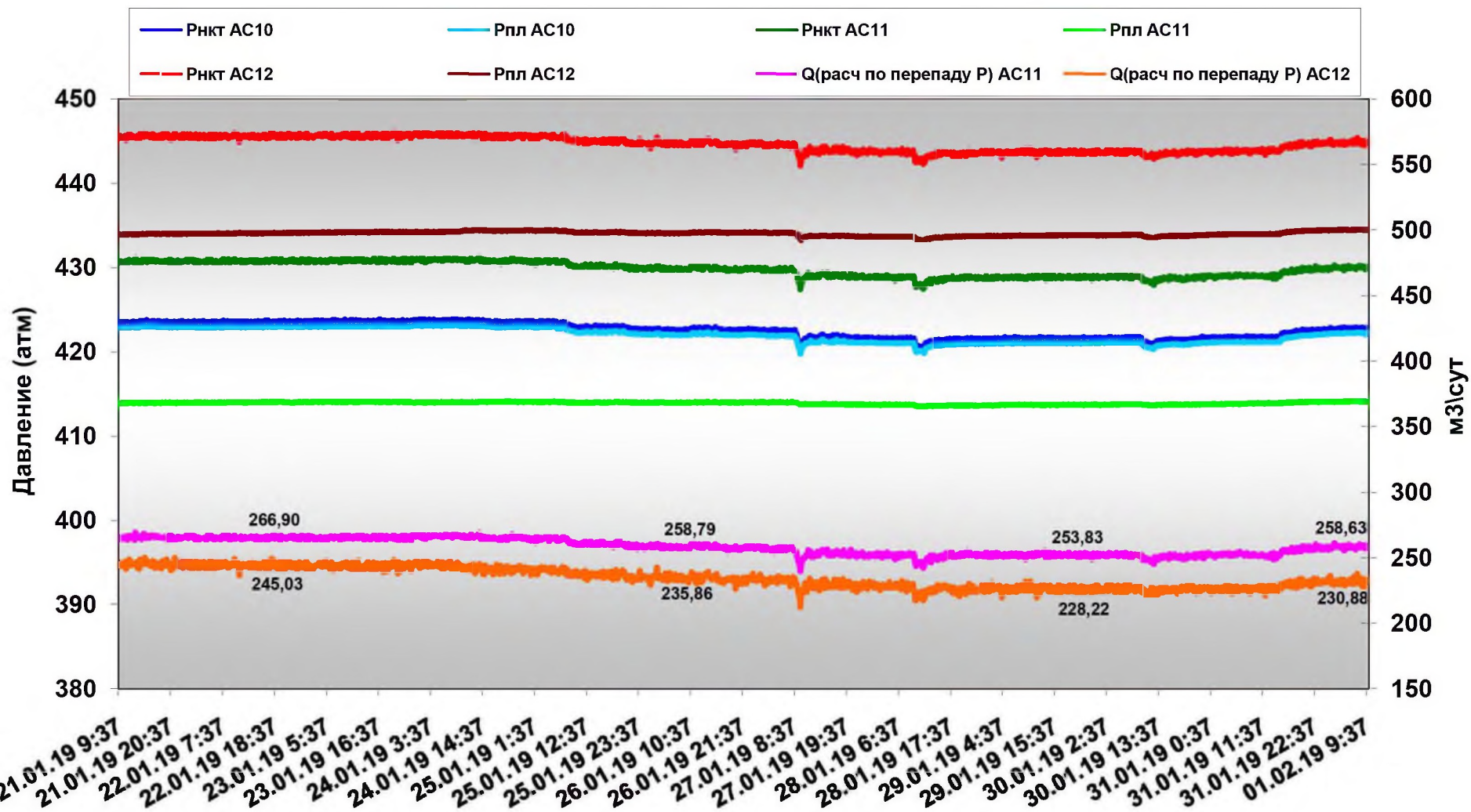
Трехпакерная компоновка с глубинным комплексом ИСДК-2G с замером давлений в режиме "on-Line" с 09ч37м 21.01.19г. по 09ч57м 01.02.19г.
