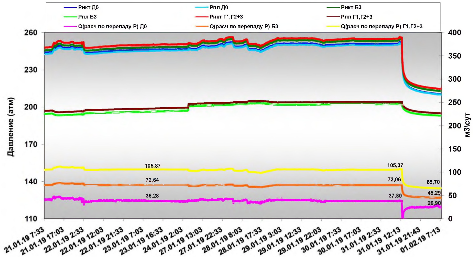
Трехпакерная компоновка с глубинным комплексом ИСДК-2G с замером давлений в режиме "on-Line" с 07ч33м 21.01.19г. по 07ч33м 01.02.19г.
