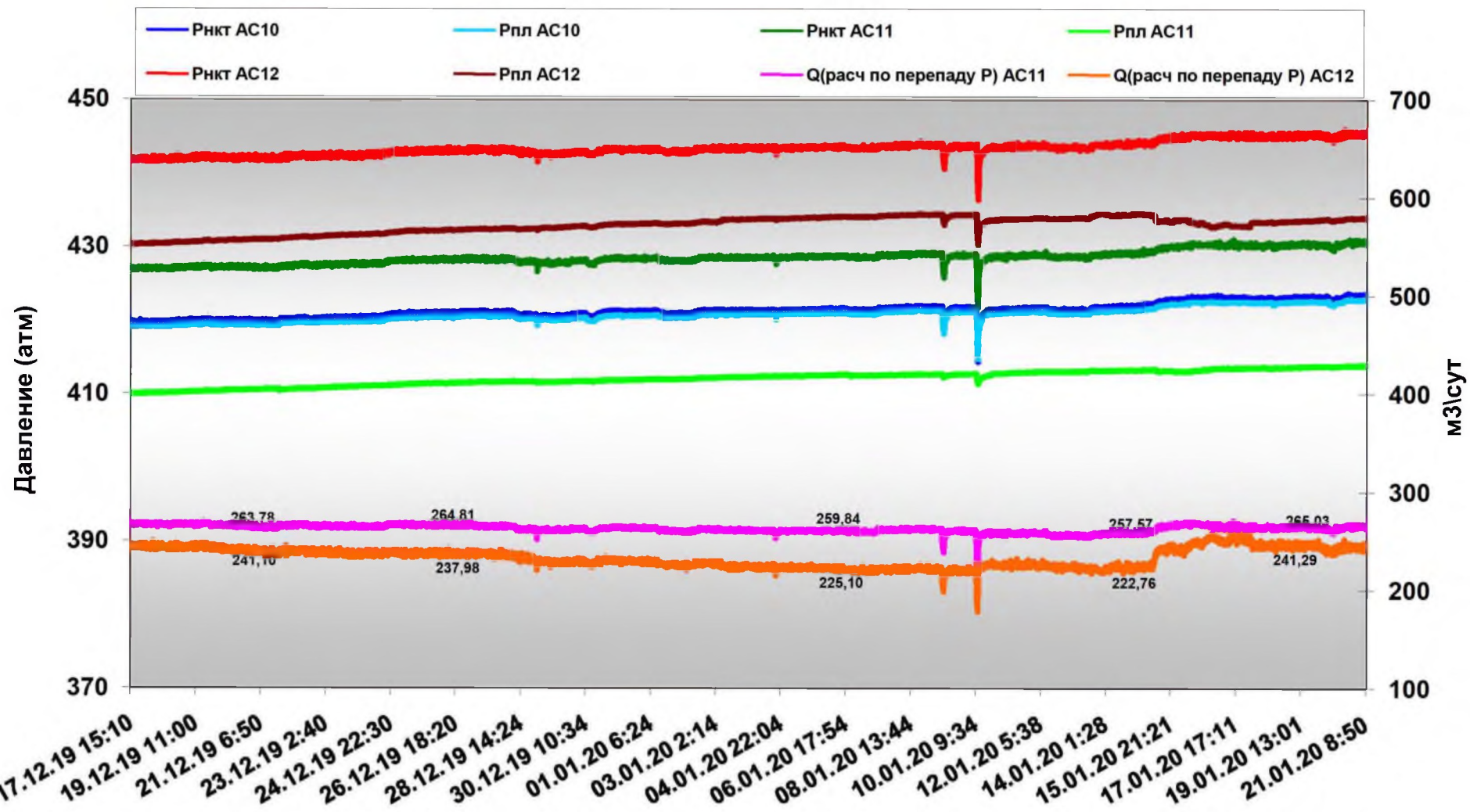
Трехпакерная компоновка с глубинным комплексом ИСДК-2G с замером давлений в режиме "on-Line" с 15ч10м 17.12.19г. по 09ч20м 21.01.20г.
